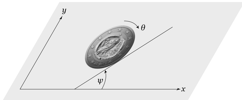
Σχήμα 4.4: Το επίπεδο του νομίσματος είναι κάθετο στο επίπεδο x - y . Το νόμισμα κυλίεται χωρίς να ολισθαίνει επάνω στο επίπεδο x - y , κινούμενο στιγμιαία στη διεύθυνση της ευθείας, η οποία σχηματίζει γωνία \psi με τον άξονα x . Κάθε σημείο στην περιφέρεια του νομίσματος προσδιορίζεται από τη γωνία \theta κατά την οποία έχει περιστραφεί συνολικά το νόμισμα καθώς κυλίεται.
