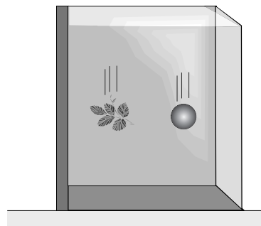
Σχήμα 4.5: Ο παρατηρητής βρίσκεται μέσα σε έναν ανελκυστήρα, ο οποίος είναι ακίνητος στην επιφάνεια της Γης. Μια μπάλα και ένα κλαδί εκτελούν ελεύθερη πτώση και επιταχύνονται προς το έδαφος με επιτάχυνση g . Υποθέτουμε ότι ο ανελκυστήρας είναι κενός και δεν υπάρχει αντίσταση.
