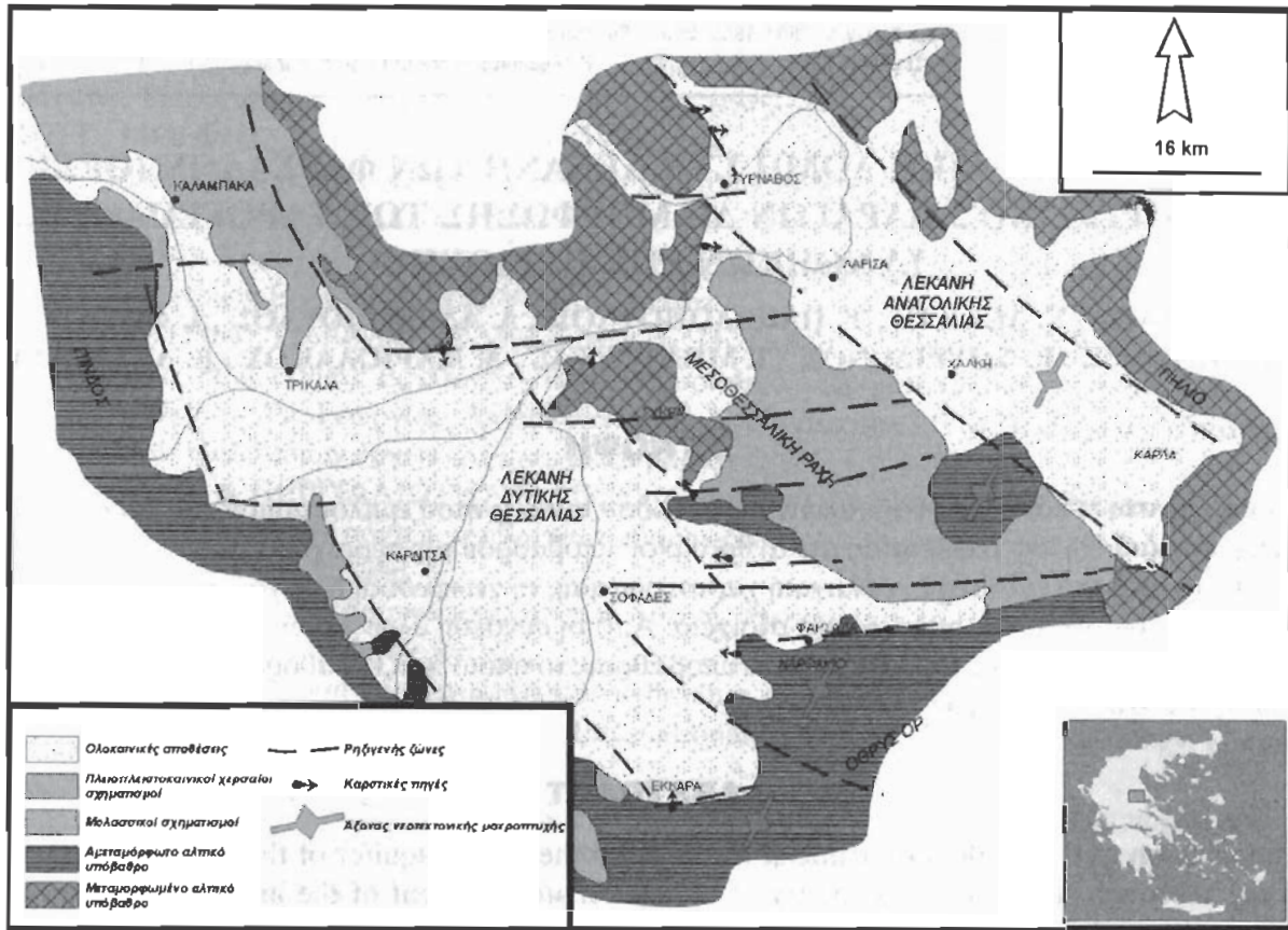
Εικόνα 1: Η περιοχή μελέτης και οι νεοτεκτονικές μακροδομές στον ευρύτερο χώρο της Θεσσαλικής λεκάνης.
