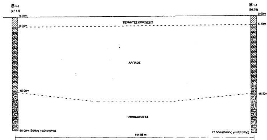
Εικόνα 2. Εδαφική τομή B1-1'EB1-3. Figure 2. Section B1-1'EB1-3.
