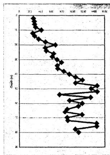
Εικόνα 6.β Κατανομή της σεισμικής ταχύτητας των εγκάρσιων κυμάτων με το βάθος.
