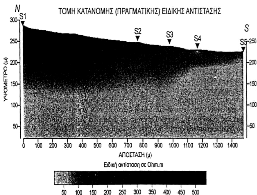
Εικόνα 4. Τομή κατανομής της (πραγματικής) ειδικής αντίστασης μετά του βάθους, σε κλίμακα 1:2. Figure 4. Resistivity cross-section, in scale 1:2.
