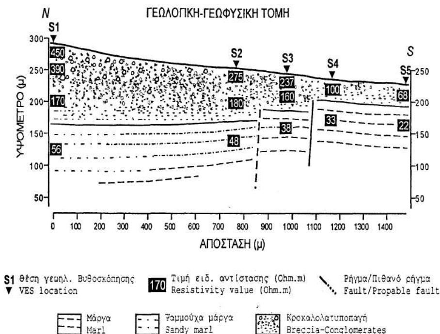
Εικόνα 5. Γεωλογική τομή, όπως προέκυψε μετά την εκτέλεση των γεωηλεκτρικών βυθοσκοπήσεων, σε κλίμακα 1:2. Figure 5. Geological section based on geophysical results, in scale 1:2.
