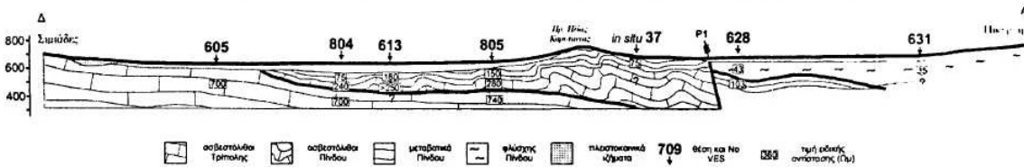
Σχήμα 5: Γεωλογική-γεωφυσική τομή A-A'.
