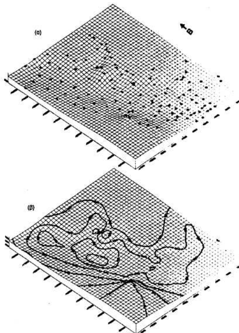
Σχήμα 4: Τρισδιάστατη απεικόνιση αναγλύφου του μορφολογικού (α) και αλπικού υποβάθρου (β), της λεκάνης της Μαντινείας, σε κλίμακα 1:1:3.
