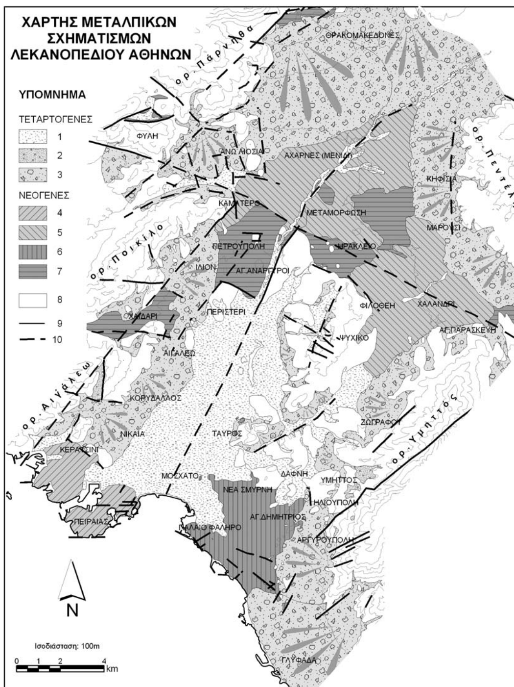
Σχήμα 1. Χάρτης μεταλπικών σχηματισμών λεκανοπεδίου Αθηνών (1. Αλλούβια, 2. Πλευρικά κορήματα, 3. Πλευρικά κορήματα και ριτίδια, 4. Πλειοκαινικοί θαλάσσιοι σχηματισμοί, 5. Πλειοκαινικοί ηπειρωτικοί σχηματισμοί, 6. Ανωμειοκαινικοί σχηματισμοί - παράκτιες και παράλιες φάσεις, 7. Ανωμειοκαινικοί ηπειρωτικοί σχηματισμοί, 8. Αλπικό υπόβαθρο, 9. Γεωλογικό όριο, 10. Ρήγμα και πιθανή προέκτασή του).
