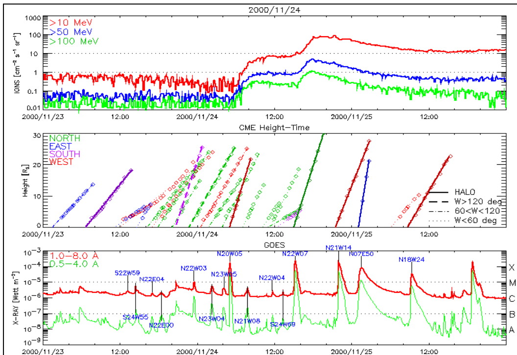
Εικόνα 3: Απεικόνιση της ροής των πρωτονίων όπως καταγράφηκαν από τους δορυφόρους GOES, των στεμματικών εκροών μάζας που καταγράφηκαν την περίοδο 23/11/2000-26/11/2000 και των αντίστοιχων ηλιακών εκλάμψεων.
