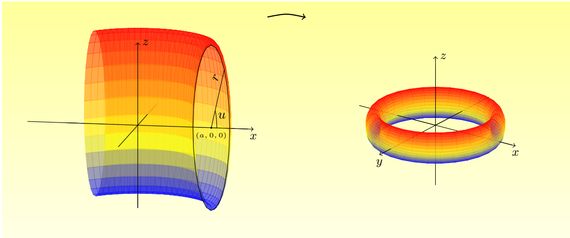
Σχήμα 2.17: Τόρος
