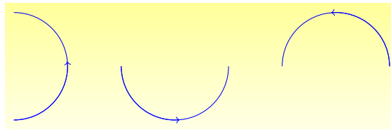
Σχήμα 1.16: Ημικύκλια ακτίνας 1
