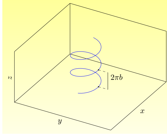
Σχήμα 1.21: Έλικοα
