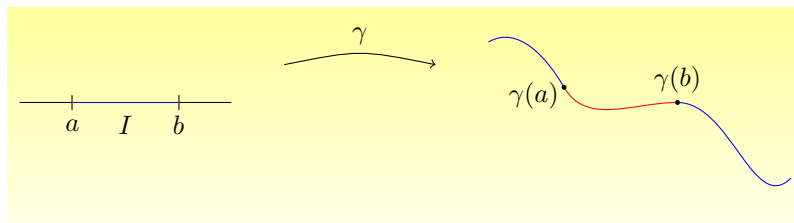
Σχήμα 1.5: Μήκος τόξου
