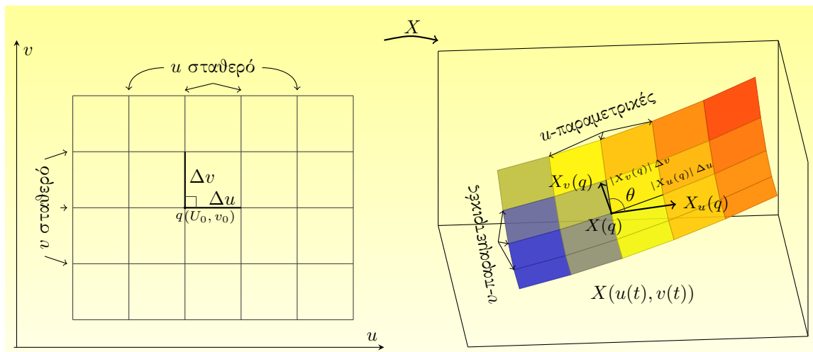
Σχήμα 2.6: Παραμετρικές καμπύλες
