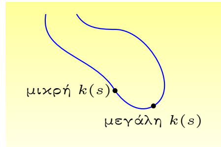
(ii) Καμπυλότητα
