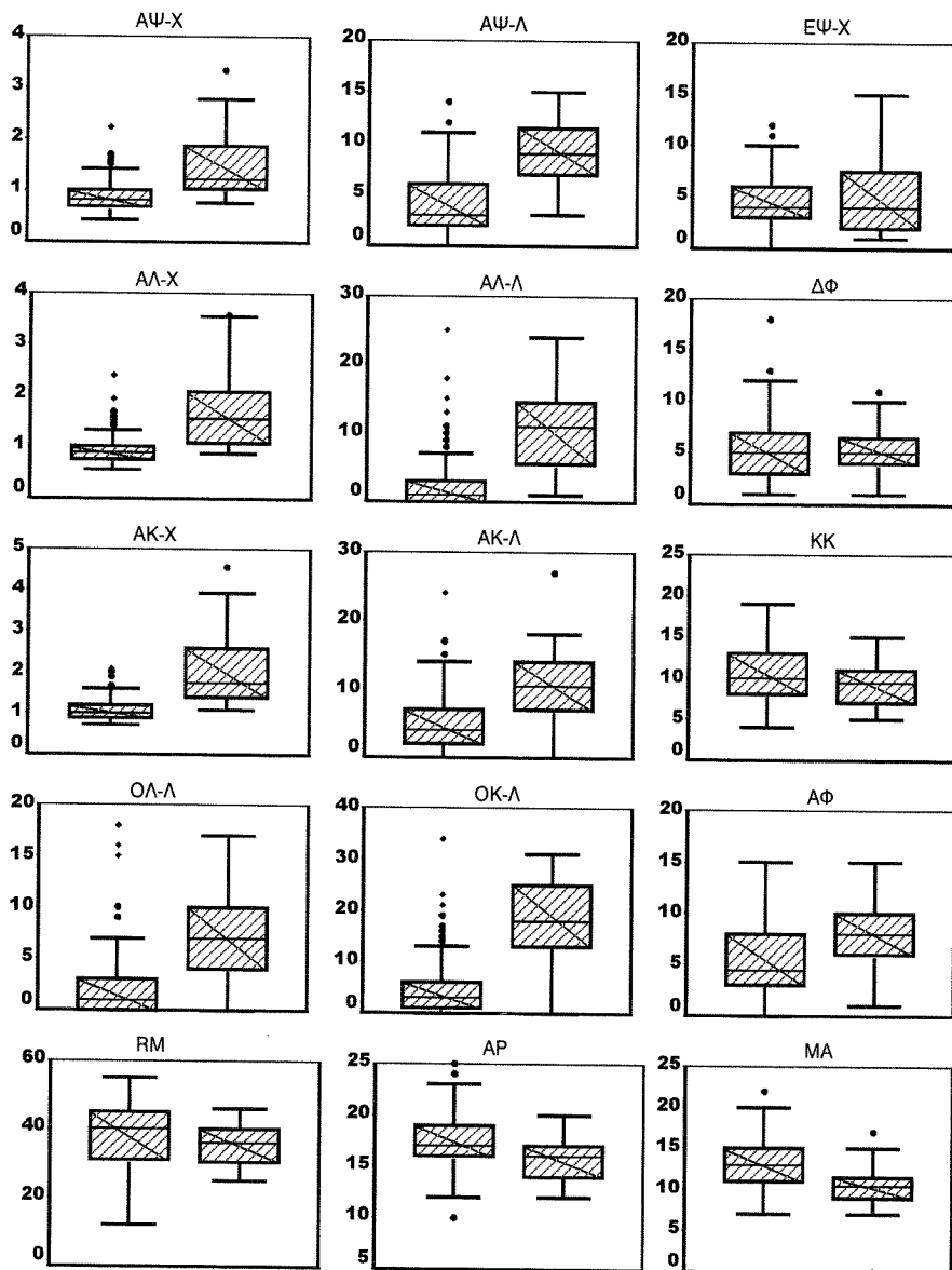
Σχήμα 1: Γραφική απεικόνιση των κατανομών ανά τεταρτημόριο από τις μετρήσεις της κλίμακας μαθησιακής αξιολόγησης στο κλινικό δείγμα (28 άτομα, αριστερά) και στο σχολικό δείγμα (137 άτομα, δεξιά). Οι ακραίες τιμές απεικονίζονται μεμονωμένα έξω από την υπόλοιπη κατανομή. Υπόμνημα: Λ=αριθμός λαθών, Χ=χρόνος. ΑΨ=ανάγνωση ψευδολέξεων, ΕΨ=επανάληψη ψευδολέξεων, ΑΛ=ανάγνωση λέξεων, ΑΚ=ανάγνωση κειμένου, ΚΚ=κατανόηση κειμένου, ΟΚ=ορθογραφία κειμένου, ΟΛ=ορθογραφία λέξεων, ΑΦ=απομόνωση φωνημάτων, RM=μήτρες Raven, ΜΑ=μήμη αριθμών, ΑΡ=αριθμητική, ΔΦ=διάκριση φθόγγων.
